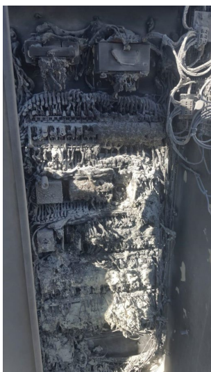
Armoire électrique
