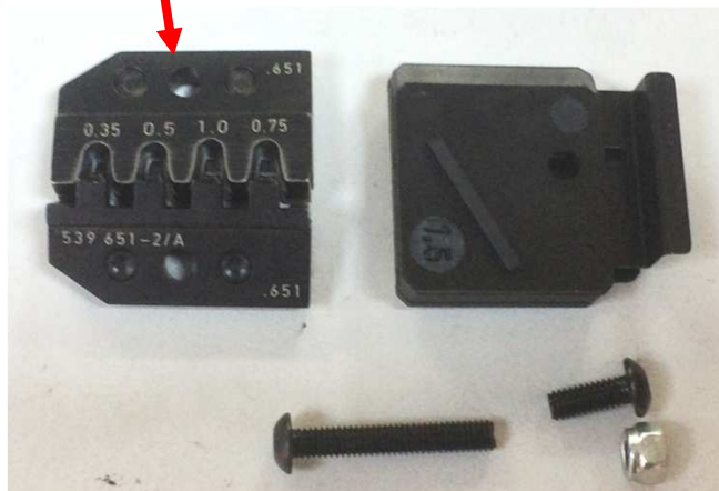
Mâchoire 84053008 Crimping die 84053008
